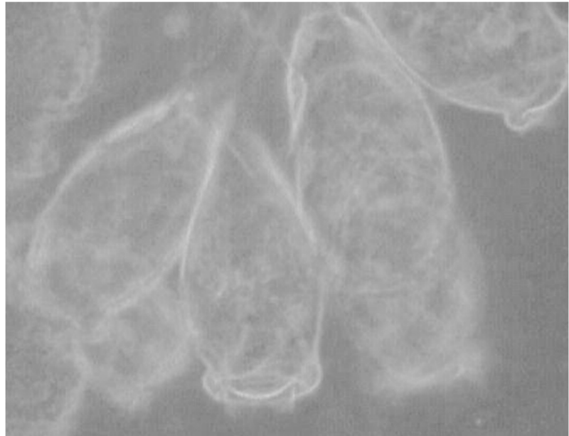
Vorticella
